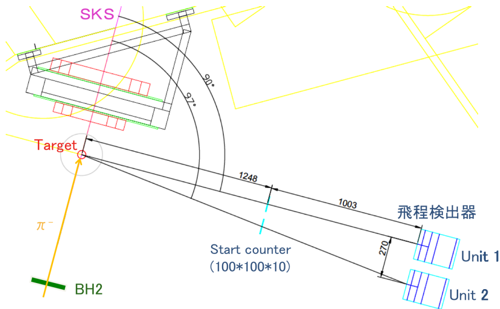
図 4.3: テスト実験のセットアップ。標的の側方 90^\circ から 97^\circ に出てくる粒子を二体の飛程検出器を用いて測定する。
