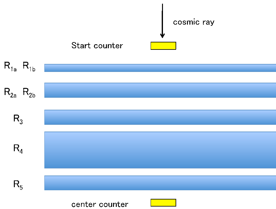
図 3.9: 宇宙線を用いた時間分解能測定のセットアップの概略図 1(宇宙線の進行方向に対して横から見た図)
