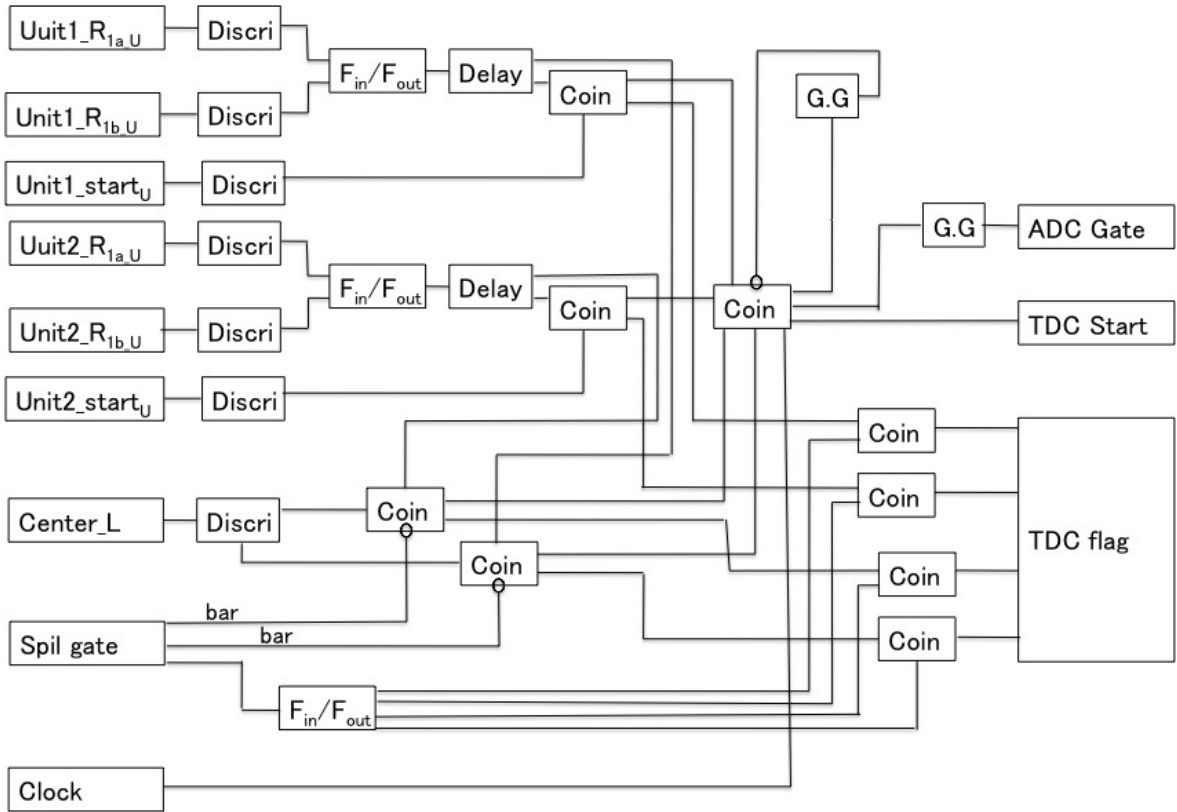
図 4.7: trigger 及びフラグに関する回路図。
