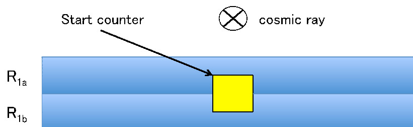
図 3.10: 宇宙線を用いた時間分解能測定のセットアップの概略図 2(宇宙線の進行方向見た図)
