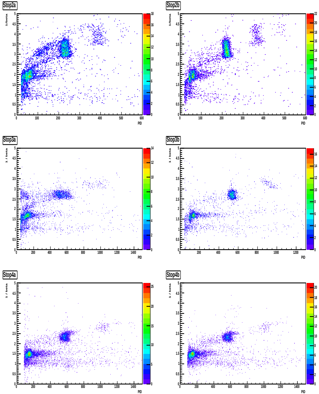
図 5.14: 各層での Stop 条件における PID と 1/\beta の相関図。それぞれの Stop 条件は (上) Stop2, (中) Stop3, (下) Stop4 であり、(左) が R_{1a} を通過したもの、(右) が R_{1b} を通過したものである。
