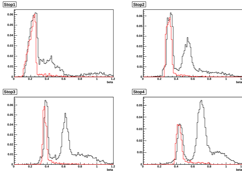
図 5.9: R_{1a} に入射した粒子に関する各層での Stop 条件における \beta の実験値とシミュレーション値の比較。それぞれ（左上）Stop1、（右上）Stop2、（左下）Stop3、（右下）Stop4 の条件下での \beta を示す。 \beta が小さいところの構造が陽子によるもので、大きい側に \pi 中間子、 \mu 粒子の構造が見られる。実験値を黒色で、陽子のシミュレーション値を赤色で示している。
