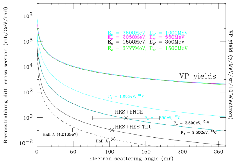
図 2.3 仮想光子起因および制動放射起因電子における散乱角のエネルギー依存性 [34]。横軸は電子の散乱角を表し、左縦軸が制動放射起因電子の断面積、右縦軸が仮想光子起因電子の断面積をそれぞれ表している。仮想光子起因電子の断面積分布が、電子ビームエネルギーの大きさに関わらず一定であるのに対し、 51 V、 12 C 標的に対して電子ビームの大きさを変えた場合の制動放射起因電子の断面積分布は大きく変化している。
