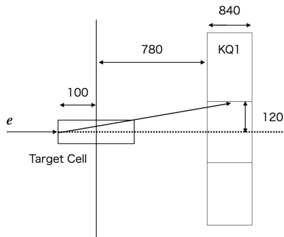
図 3.4 Target Cell の高さ議論のための概略図
